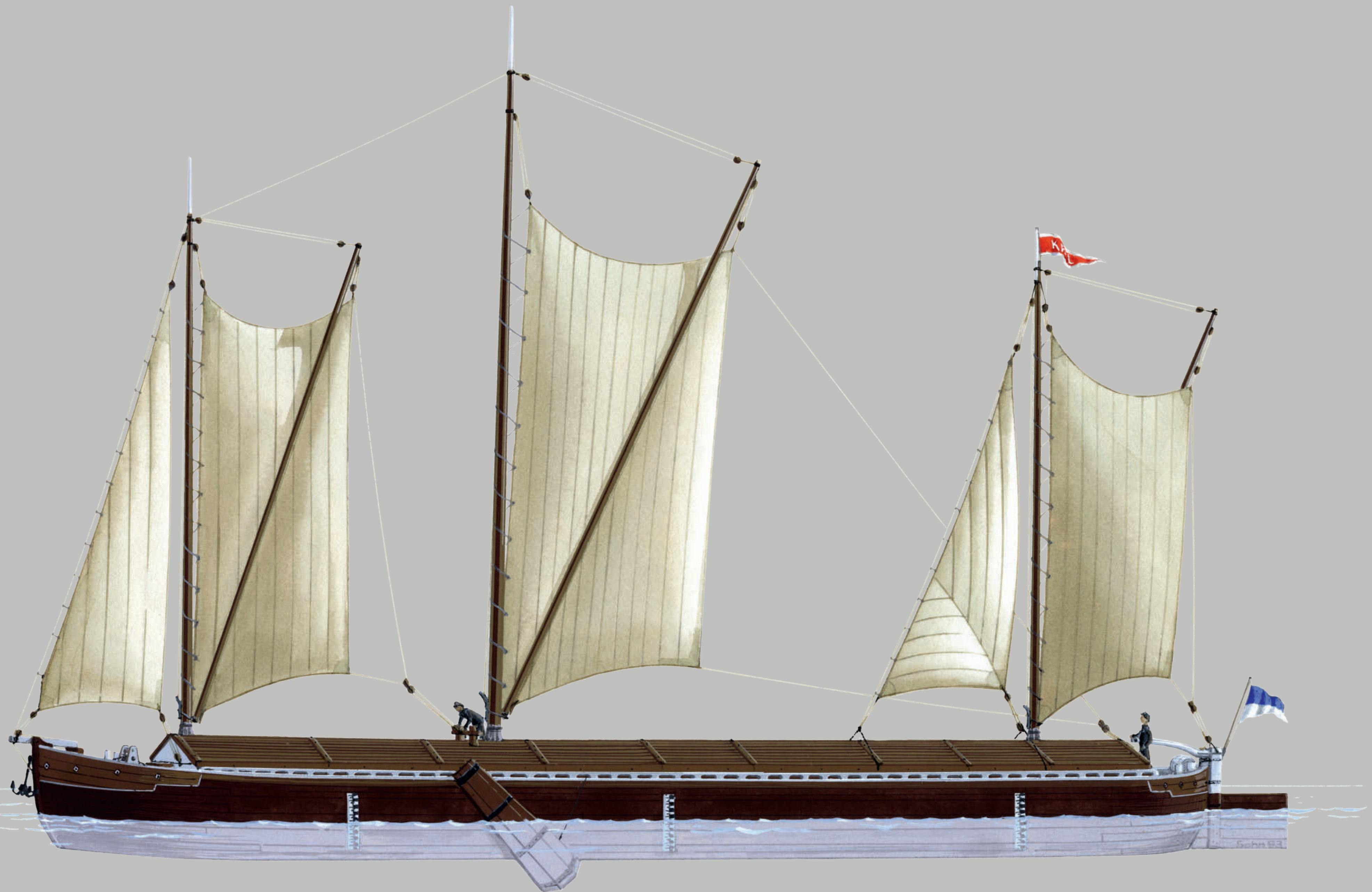
POMMERSCHER MOLLENKAHN UM 1925
