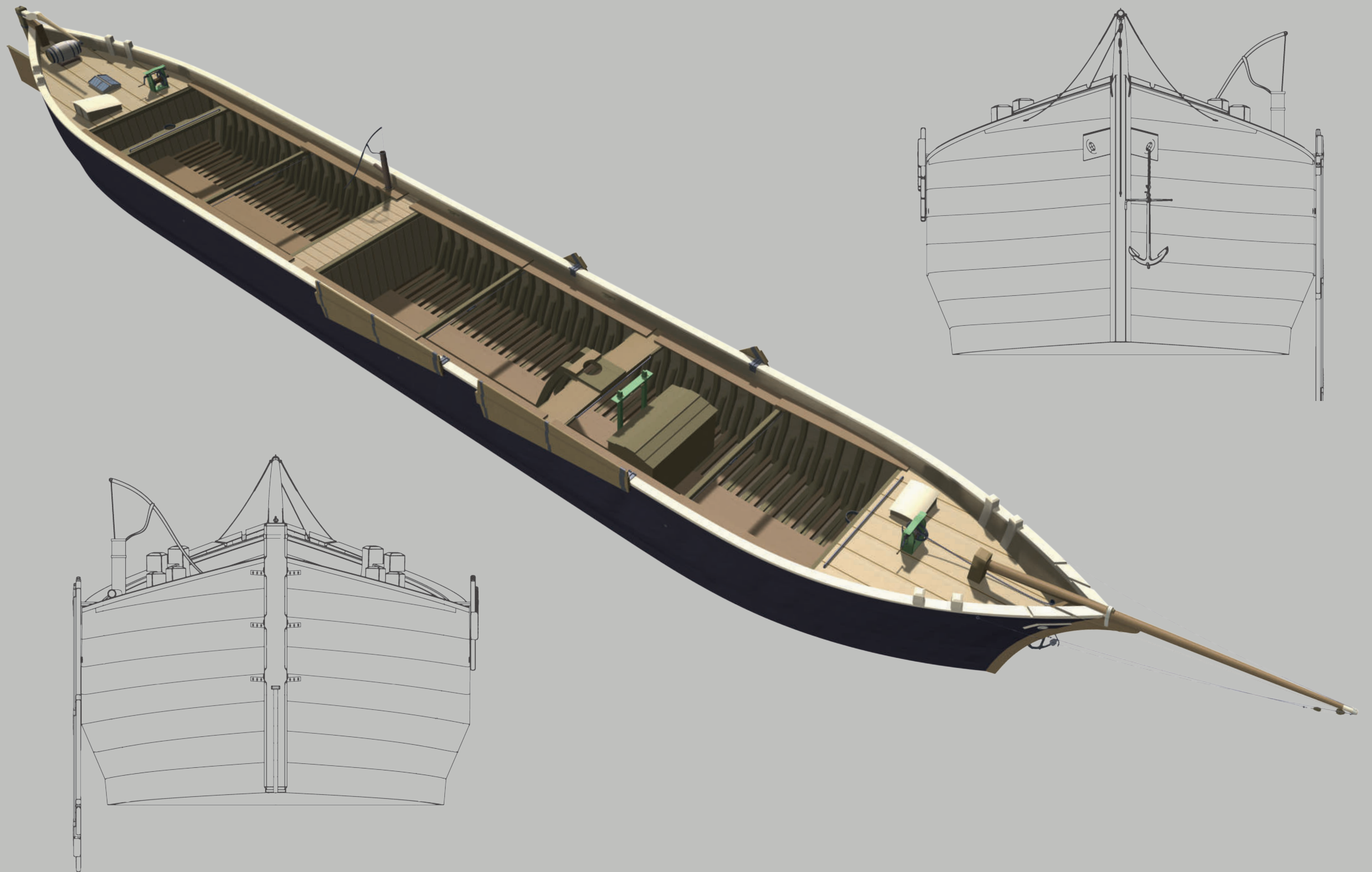
POMMERSCHER STEVENKAHN UM 1915
