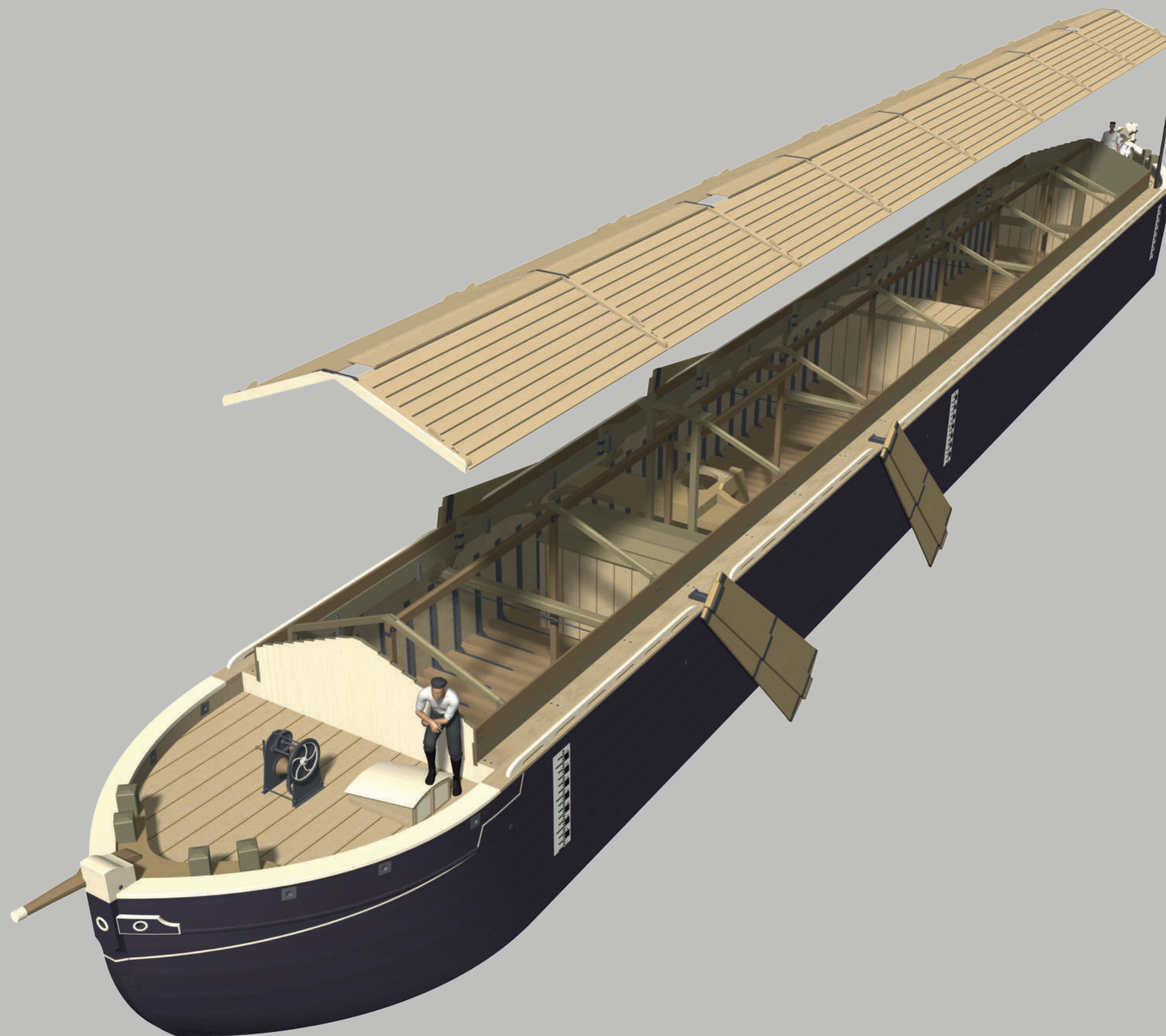
POMMERSCHER MOLLENKAHN UM 1925
